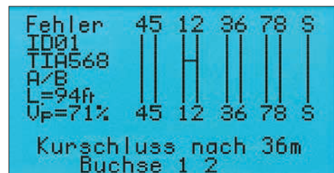
ID01 weist auf einen Kurzschluss im Paar 1-2 des mit dem Identifizierer Nr.1 endenden Kabels hin
